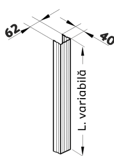
② Profil metallic de fixare pe stâlp 60
