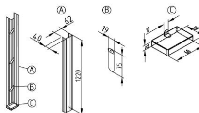
profil de fixare pe stâlp click-fix 60 X121, 2F
