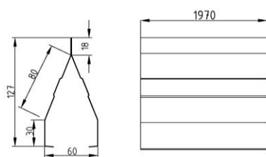
capac închidere 60 gard orizontal X121, 2F
