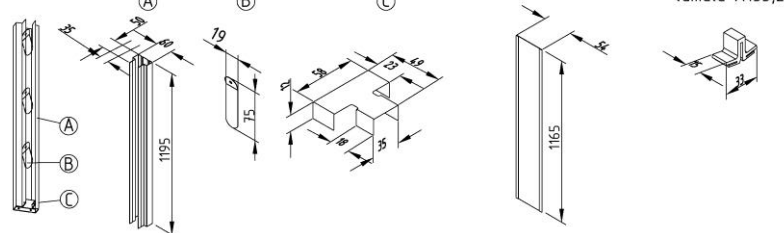
profil de fixare pe stâlp click-fix 35 X135,2F platbandă aliniere distanțiere HDPE lamele X135,2F
