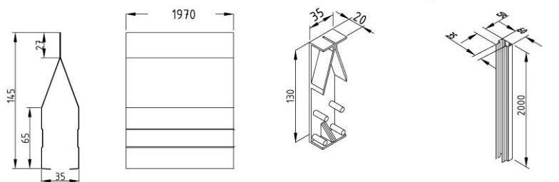
profil de fixare pe stâlp click-fix 35 X135,2F platbandă aliniere distanțiere HDPE lamele X135,2F
