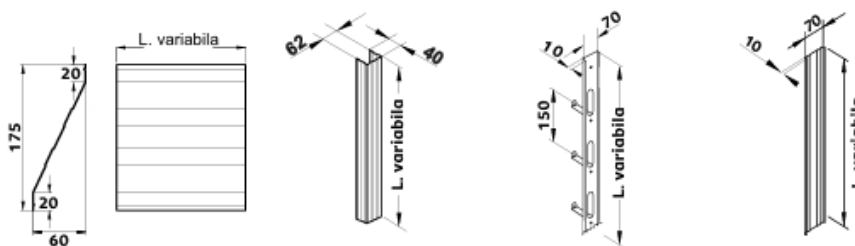
① Lamela front 170 ② Capac închidere 60 ③ Rigla rigidizare ④ Capac rigla rigidizare
