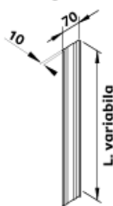
⑤ Capac rigla rigidizare
